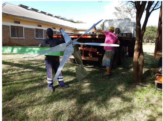
Fig.7: Operazioni di montaggio di un generatore eolico
